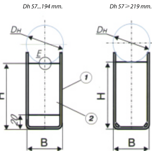
Опора для трубопрово- дов без спутника
